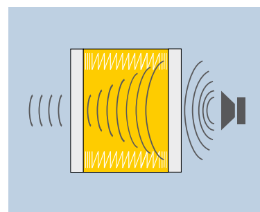
Princip dušenja zvoka suhomontažne stene: masa - vzmet - masa
