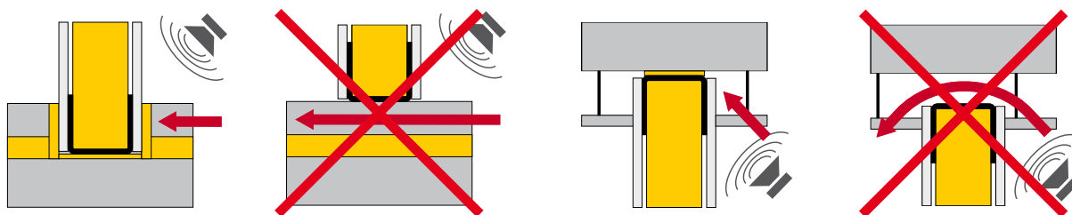
Pravilna in nepravilna postavitev stene na tla s plavajočim estrihom
